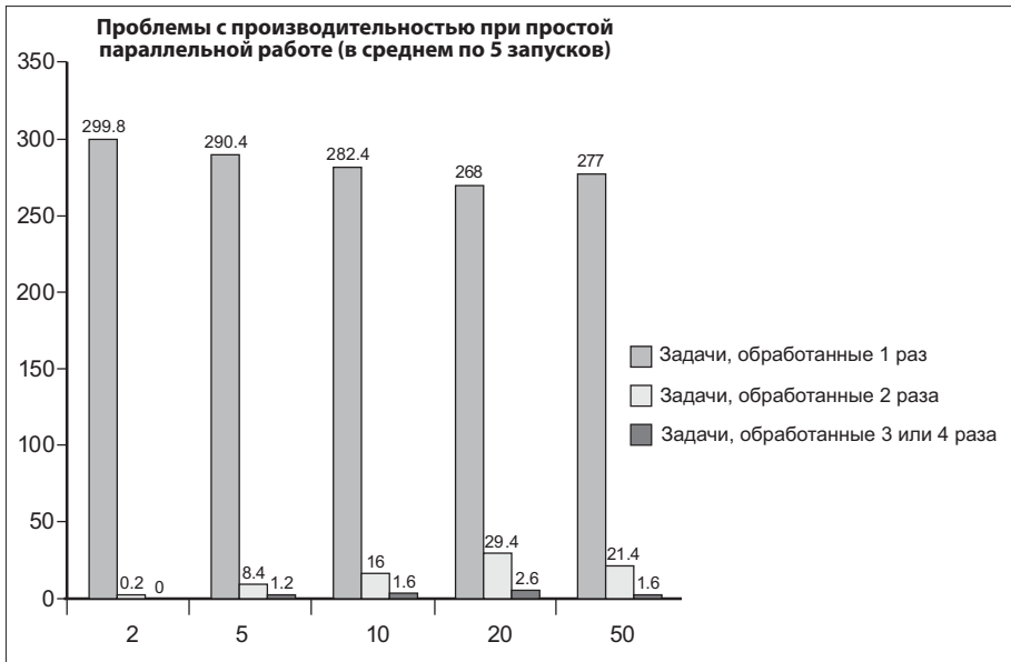
Рис. 7.2. Когда конкуренция приводит к печальным последствиям
