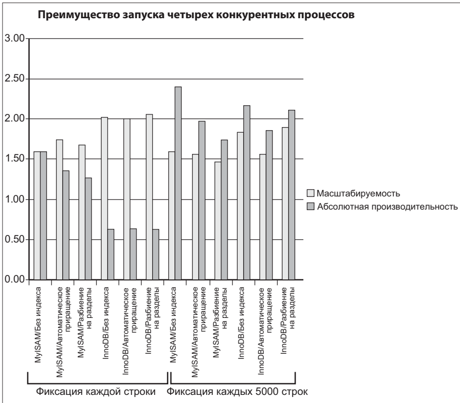
Рис. 7.7. Сравнение производительности и масштабируемости с четырьмя процессами
