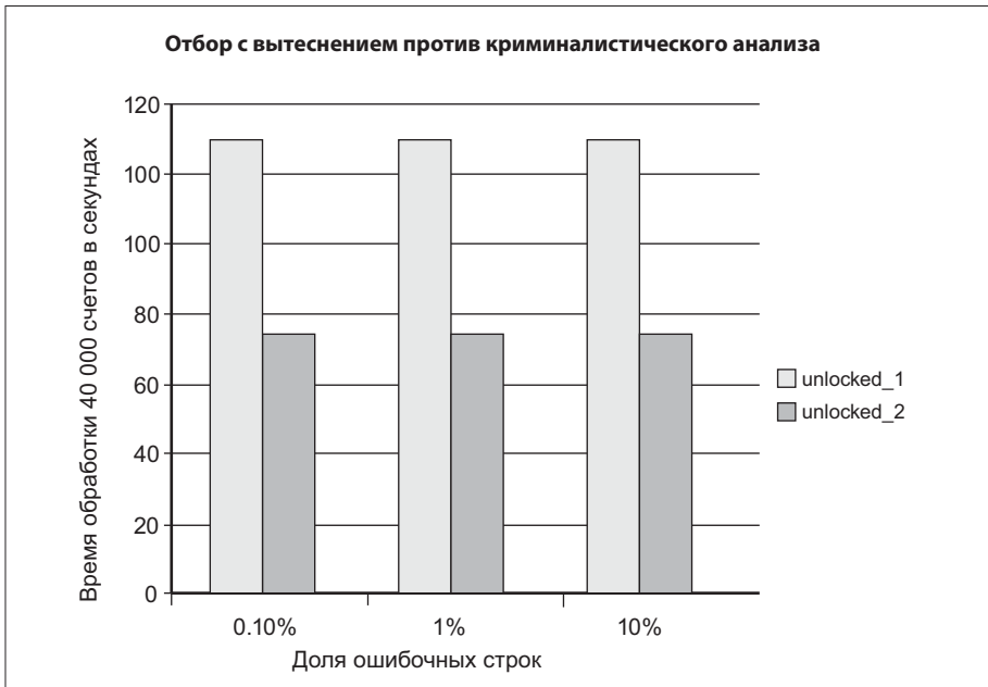
Рис. 6.1. Функция, которая проверяет и делает, в сравнении с функцией, которая делает и проверяет (SQL Server/Visual Basic)
