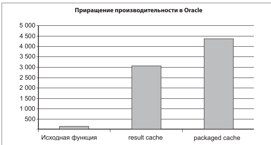
Рис. 3.4. Сравнение альтернативных способов написания функции преобразования валюты в Oracle
