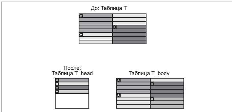
Рис. 7.10. Разбиение таблиц
